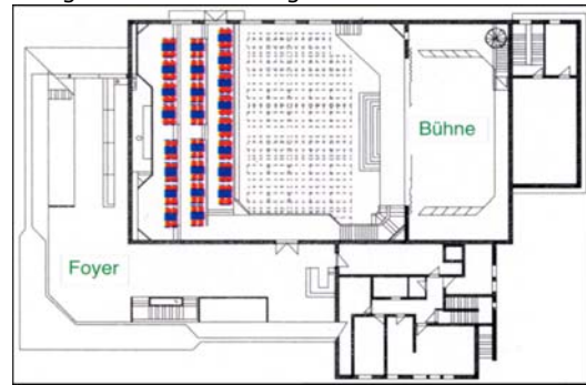
Obergeschoß Bestuhlungsvariante 2
